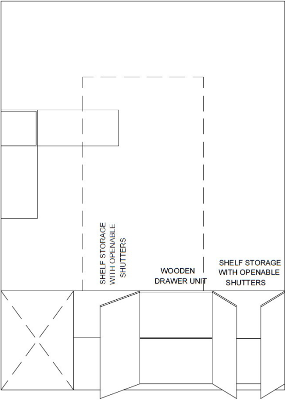
ELEVATION ②
